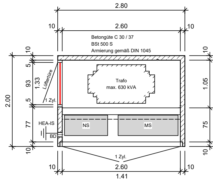
GRUNDRISS
