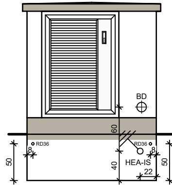
Ansicht
