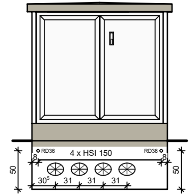
Ansicht
