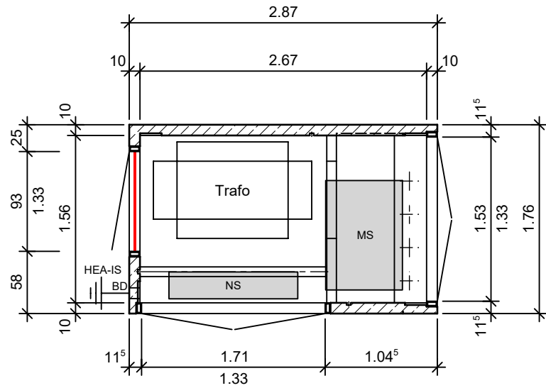
Grundriss
