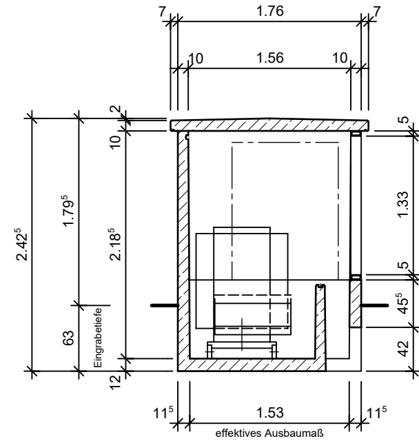
Schnitt
