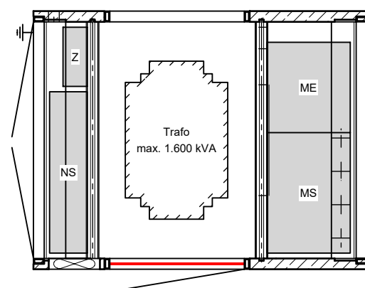
W3124 bis 1.600 kVA
