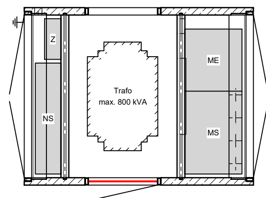
W3124 bis 800 kVA
