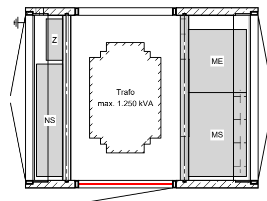
W3124 bis 1.250 kVA
